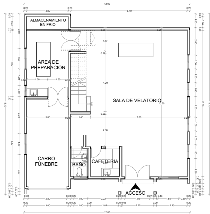
PLANTA ARQUITECTÓNICA DIMENSIONADA ESC. 1:100 PRIMER NIVEL AREA: 138 M 2
