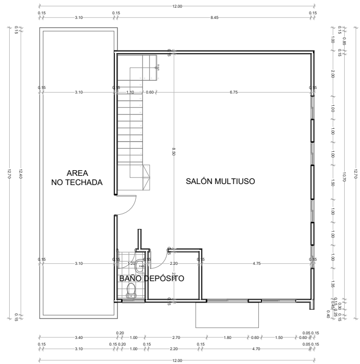
PLANTA ARQUITECTÓNICA DIMENSIONADA ESC. 1:100 SEGUNDO NIVEL AREA: 96 M 2
